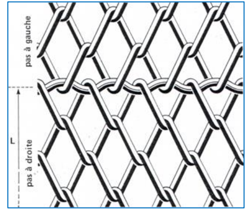
Montage en panneaux inversés avec tringles
